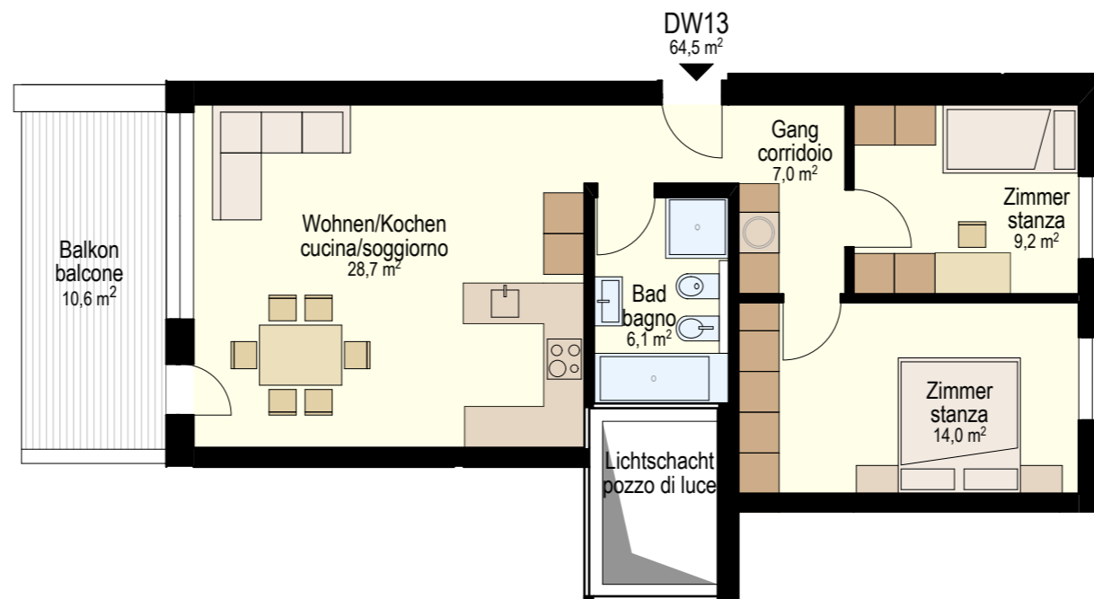
4. OBERGESCHOSS - PIANO QUARTO DW13 Maßstab - scala 1:100 ➤ N
