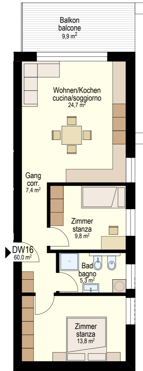
4. OBERGESCHOSS - PIANO QUARTO DW16 Maßstab - scala 1:100 ➤ N
