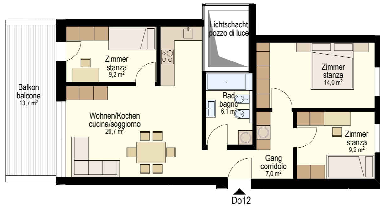
3. OBERGESCHOSS - PIANO TERZO Do12 Maßstab - scala 1:100 ➤ N
